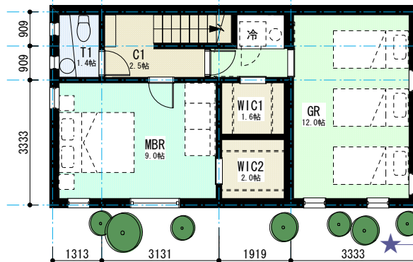
半地下階平面図 scale 1:100
