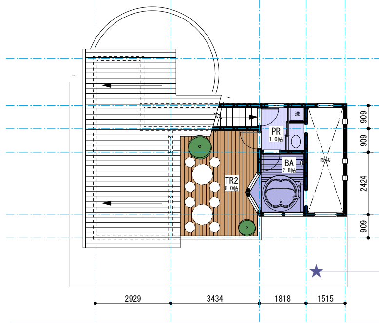
2階平面図 scale 1:100
